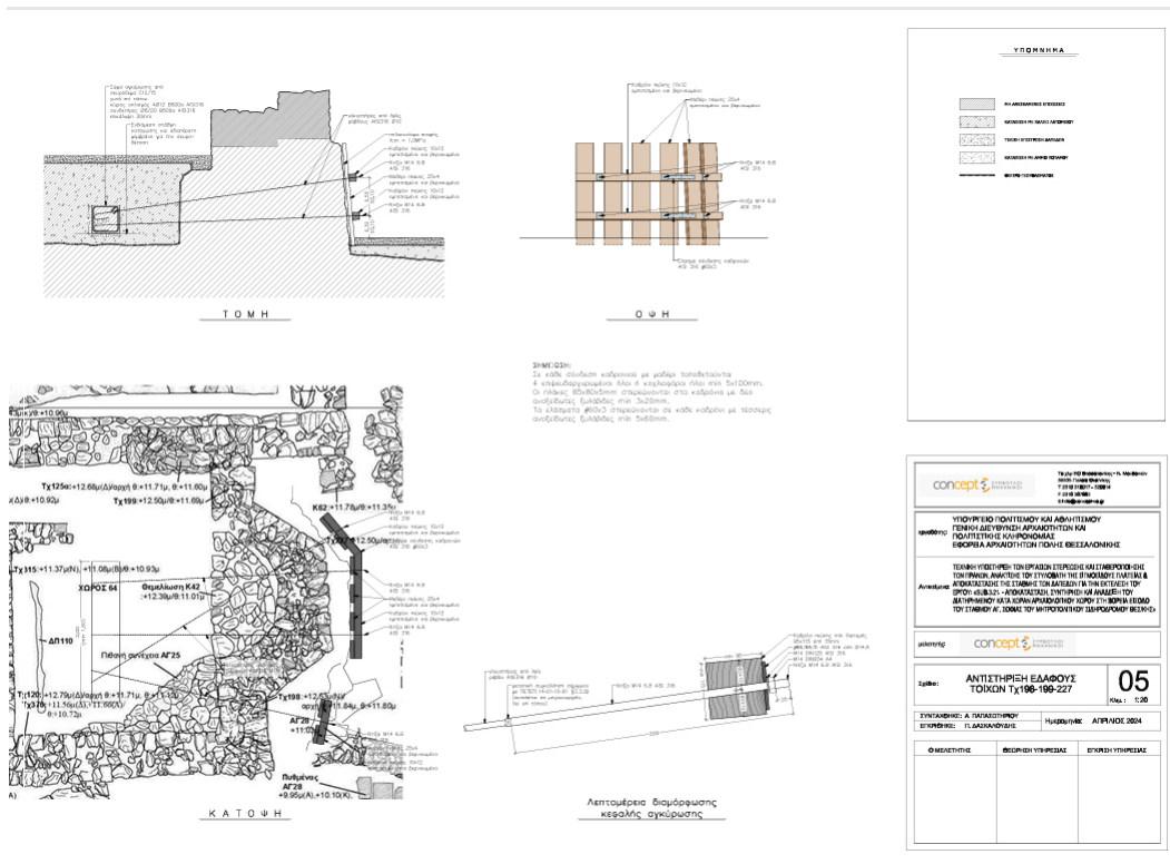
σχ.05. Αντιστήριξη εδάφους τοίχων Τχ198, Τχ227, Τχ199
