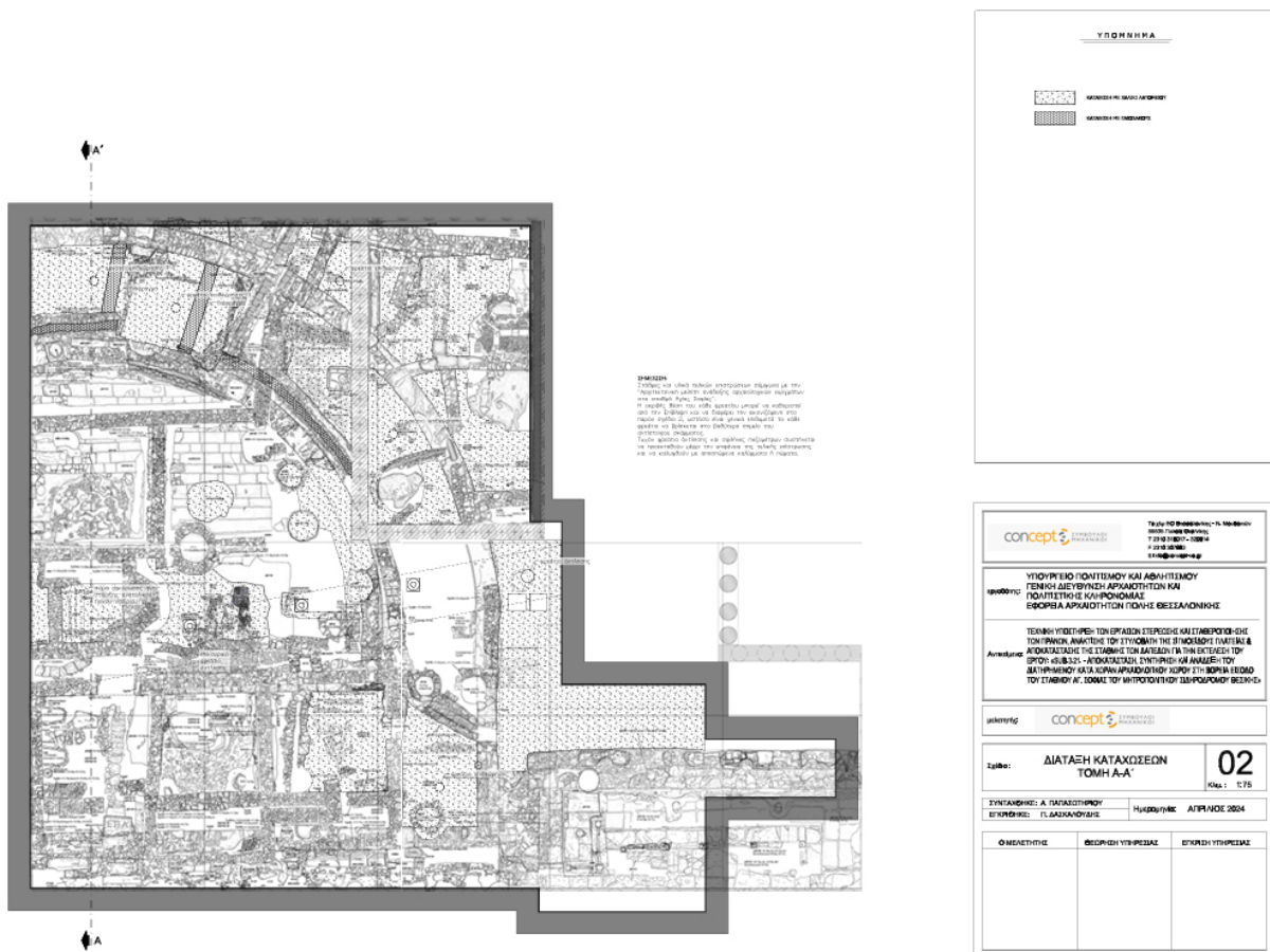
σχ.02. Διάταξη καταχώσεων
